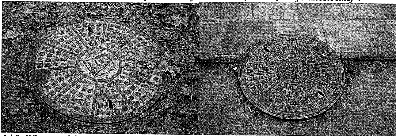
1 i 2. Włazy studzienek rewizyjnych Ø1000 na sieci kanalizacji sanitarnej
